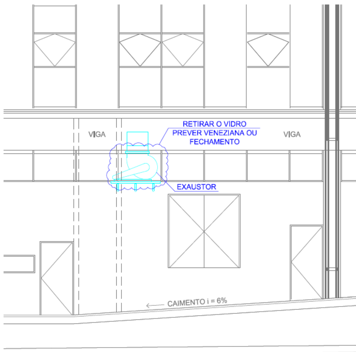
VISTA 01 ESC.: 1:50
