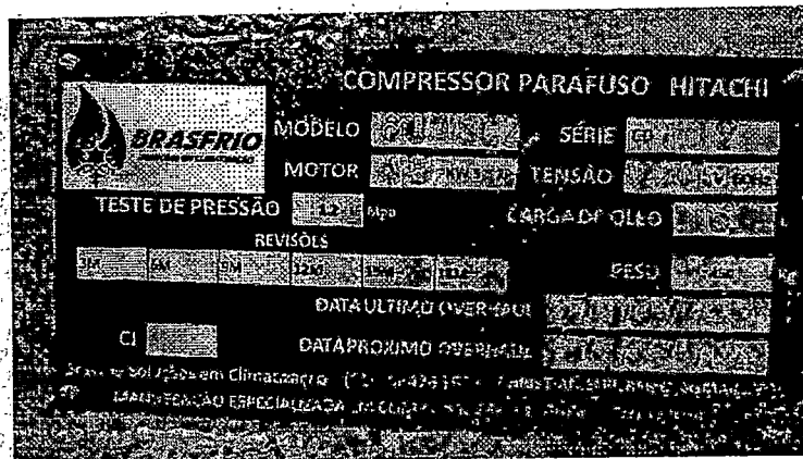
Nova placa de identificação do compressor.
