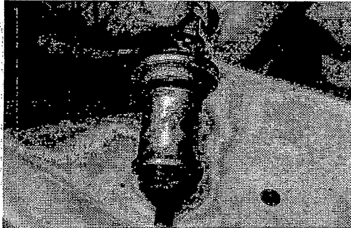
Agulha da válvula de expansão substituída totalmente contaminada e desgastada.
