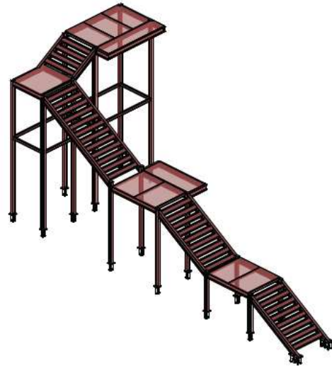
Degrau Típico - Escada 1
