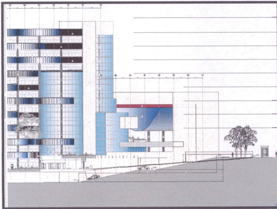
FACHADA D – TRECHO 2
