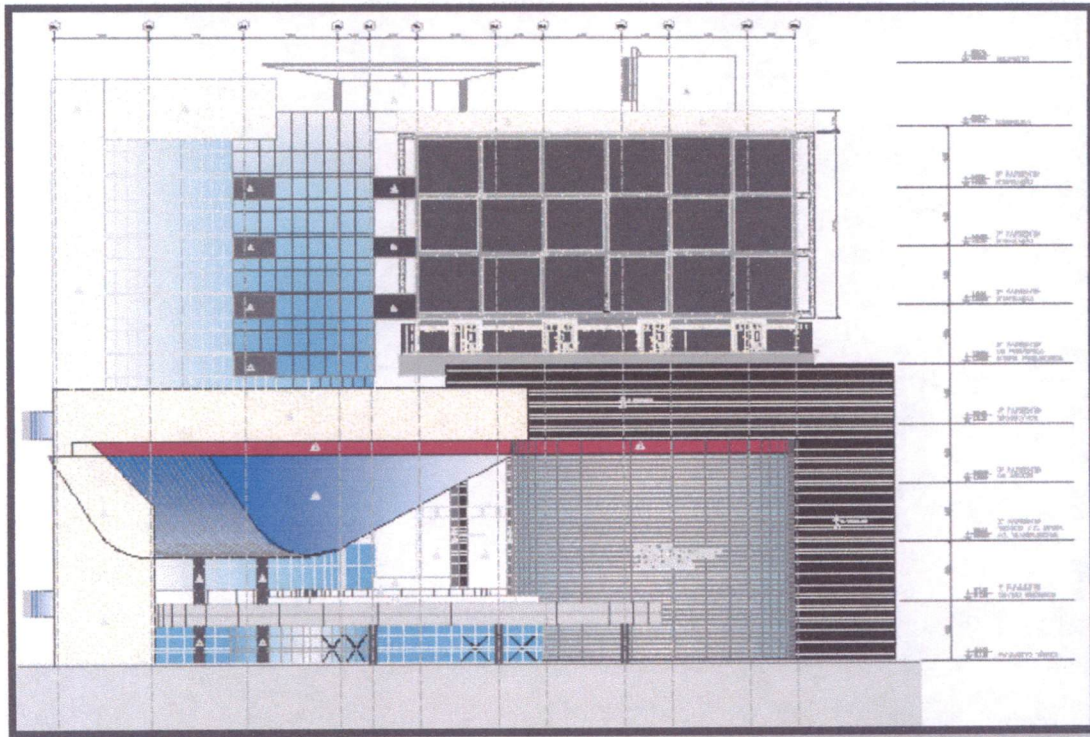
FACHADA A
