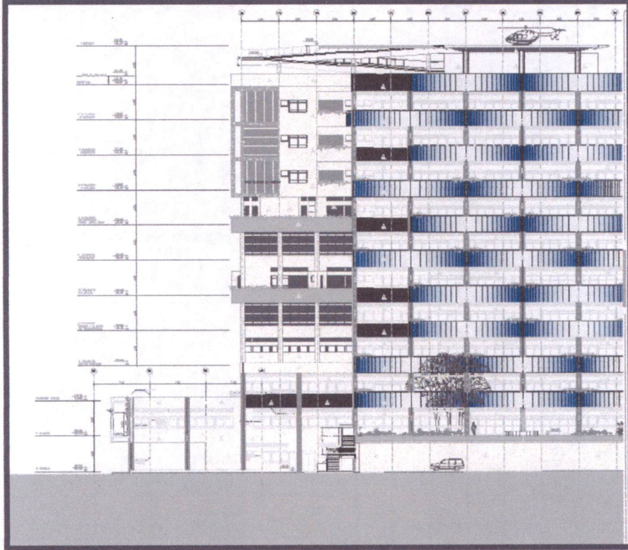
FACHADA D – TRECHO 1
