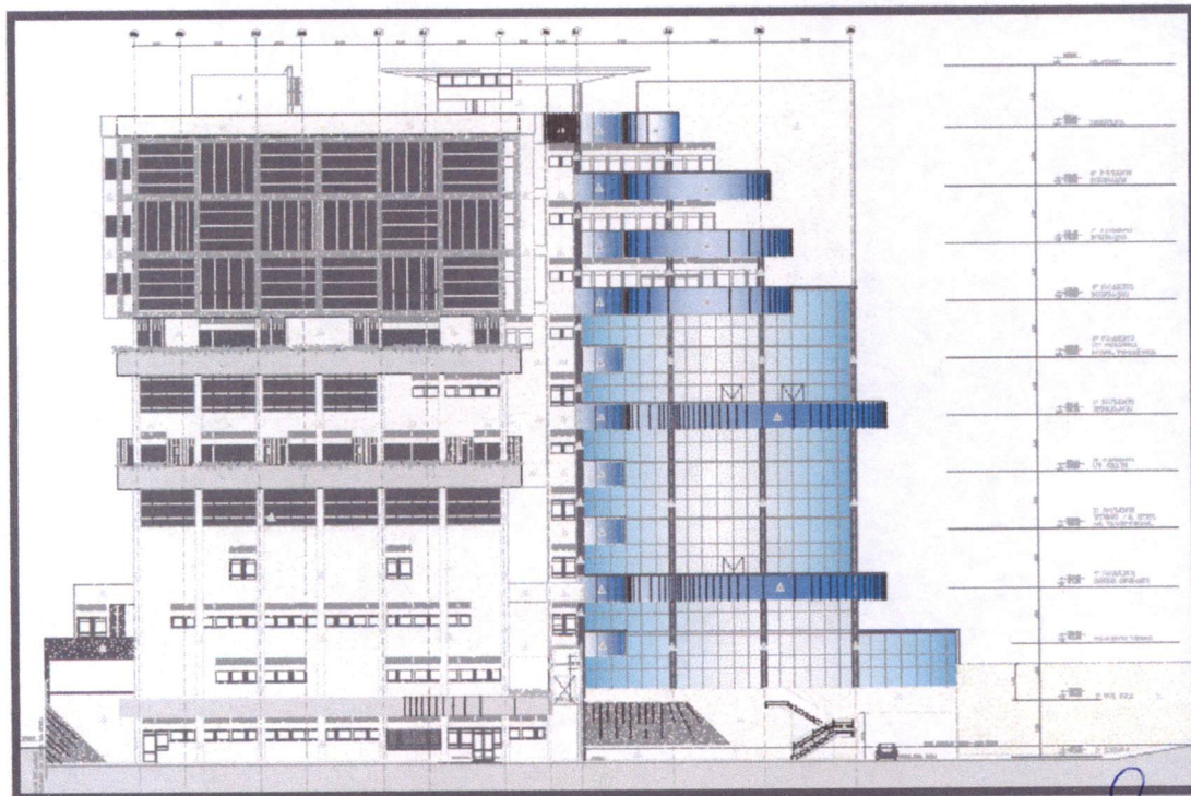
FACHADA B
