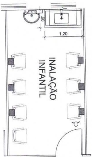
SALA DE INALAÇÃO INFANTIL - PLANTA BAIXA ESC. 1.25
