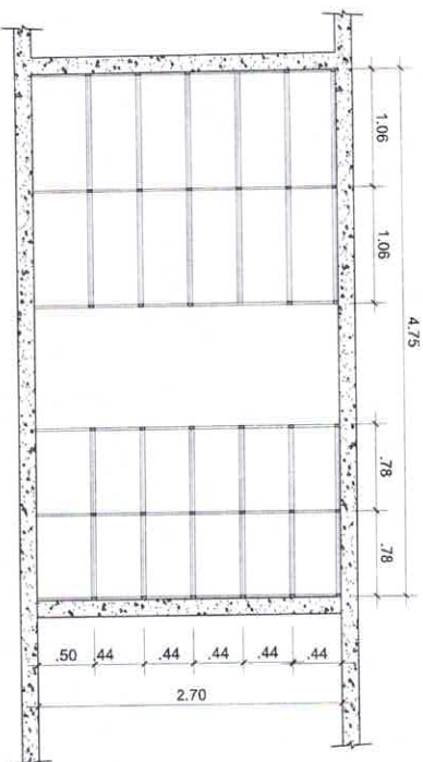
ESTRUTURA METÁLICA PARA PASTA DE SUSPENSÃO - VISTA A ESC. 1/25
