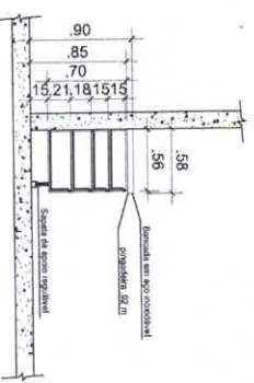
GABINETE PLANEJADO - VISTA C ESC. 1.25
