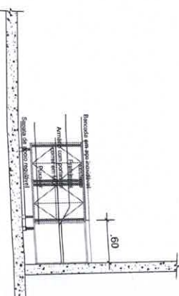
GABINETE PLANEJADO - VISTA D ESC. 1/25
