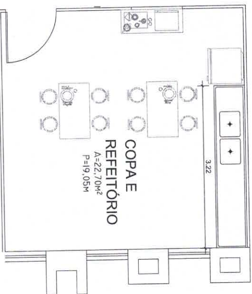
COPA - REFEITÓRIO - (PLANTA BAIXA) ESC. 1/25
