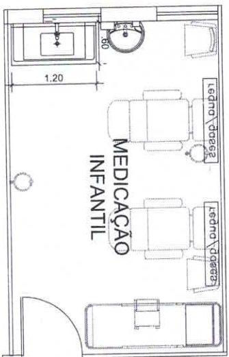
SALA DE MEDICAÇÃO INFANTIL - PLANTA BAIXA ESC. 1,25
