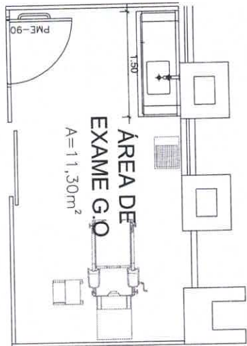
SALA DE G.O. (ÁREA DE EXAME) - PLANTA BAIXA
