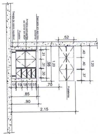
GABINETE PLANEJADO E ARMÁRIO SUSPENSO - VISTA A ESC. 1/25
