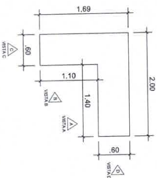
PIA EM AÇO INOX EXISTENTE - (PLANTA BAIXA) ESC. 1/25
