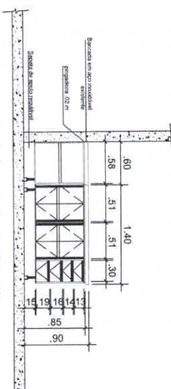
GABINETE PLANEJADO - VISTA A ESC. 1/25
