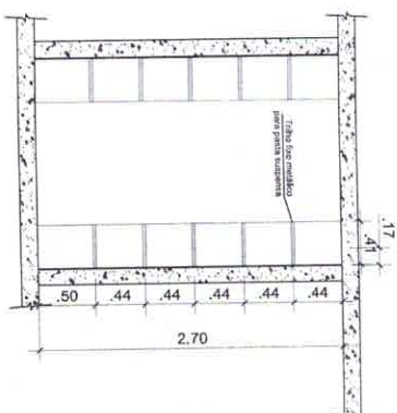
ESTRUTURA METÁLICA PARA PASTA DE SUSPENSÃO - VISTA B ESC. 1/25
