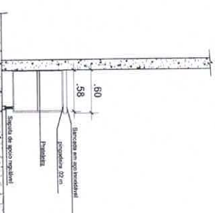
GABINETE PLANEJADO E ARMÁRIO SUSPENSO - VISTA C ESC. 1.25
