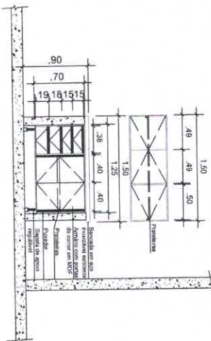
GABINETE PLANEJADO E ARMÁRIO SUSPENSO - VISTA A ESC. 1,25
