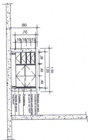
GABINETE PLANEJADO E ARMÁRIO SUSPENSO - VISTA A ESC. 1/25
