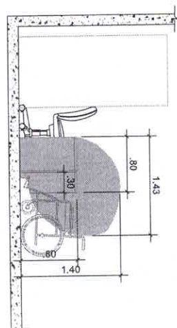
BALÇÃO DE ATENDIMENTO - (VISTA C) Esc: 1,28
