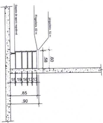
GABINETE PLANEJADO E ARMÁRIO SUSPENSO - VISTA B ESC. 1,25
