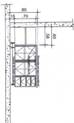
GABINETE PLANEJADO - VISTA C ESC. 1/25
