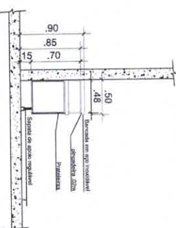
GABINETE PLANEJADO - VISTA C ESC. 1,25
