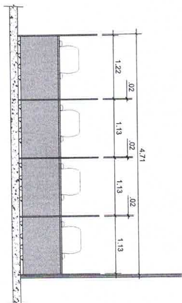
BALÇAO DE ATENDIMENTO - (VISTA B) ESC 173
