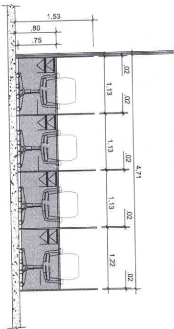
BALÇÃO DE ATENDIMENTO - (VISTA A)
