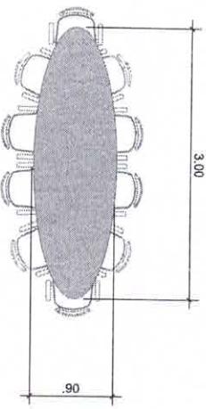
MESAS DE ESCRITÓRIO OVAL 10 LUGARES - TIPO PADRÃO - PLANTA BAIXA ESC. 1:25
