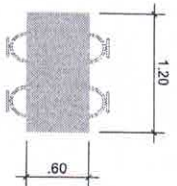
MESA DE REFETÓRIO 4 LUGARES - TIPO PADRÃO - PLANTA BAIXA ESC. 1:25
