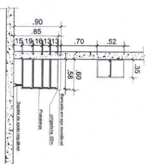
GABINETE PLANEJADO E ARMÁRIO SUSPENSO - VISTA B ESC. 1.25
