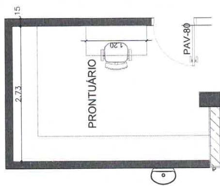
PRONTUÁRIO DA RECEPÇÃO - (PLANTA BAIXA) ESC. 1:25
