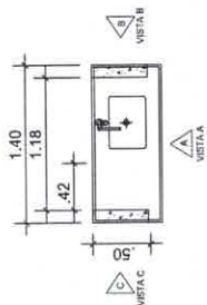
PIA EM AÇO INOX EXISTENTE - (PLANTA BAIXA) ESC. 1.25
