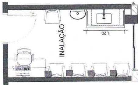
PIA EM AÇO INOX EXISTENTE - (PLANTA BAIXA) ESC. 1:25
