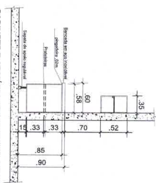
GABINETE E ARMÁRIO SUSPENSO PLANEJADO - VISTA B ESC. 1.25
