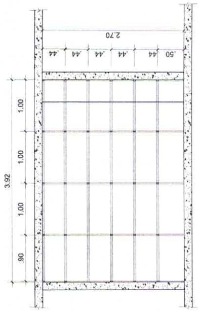
ESTRUTURA METÁLICA PARA PASTA DE SUSPENSÃO - VISTA A ESC. 1:25
