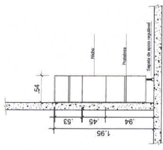
GABINETE PLANEJADO E ARMÁRIO SUSPENSO - VISTA B ESC. 1:25
