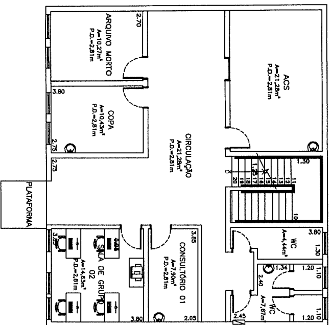
UBS JARDIM TIETÊ II - PLANTA PAV. SUPERIOR
